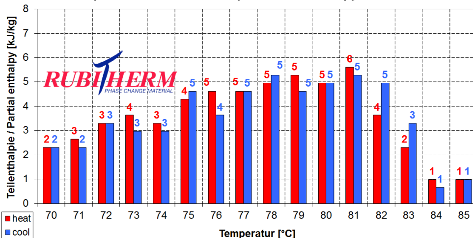
Beispiel: GR82 1-3 Teilenthalpie / Partial enthalpy distribution
