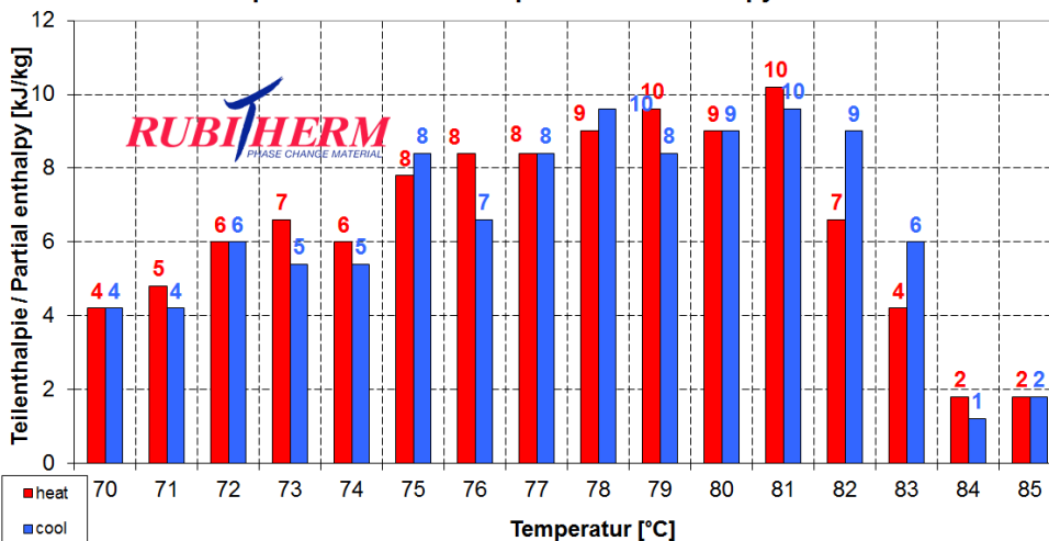
Beispiel: PX82 Teilenthalpie / Partial enthalpy distribution
