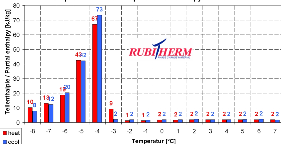
Beispiel: RT- 4 Teilenthalpie / Partial enthalpy distribution
