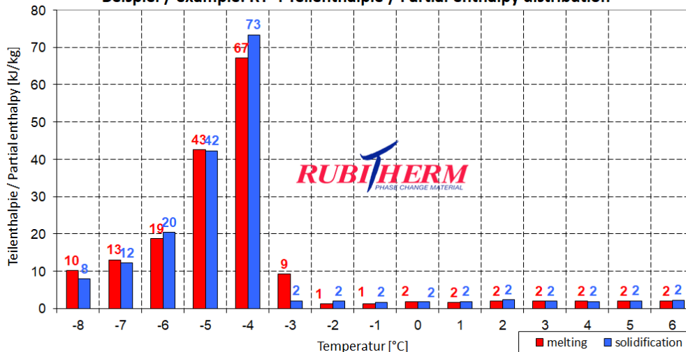
Beispiel / example: RT-4 Teilenthalpie / Partial enthalpy distribution
