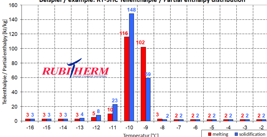
Beispiel / example: RT-9HC Teilenthalpie / Partial enthalpy distribution
