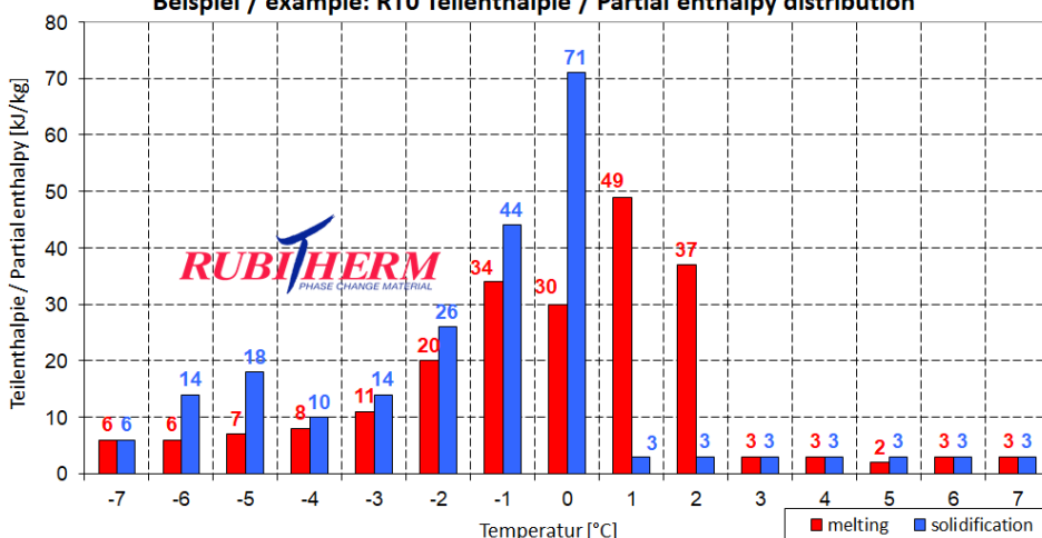
Beispiel / example: RT0 Teilenthalpie / Partial enthalpy distribution
