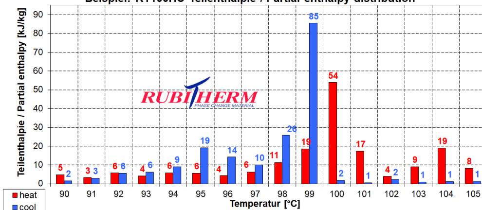
Beispiel: RT100HC Teilenthalpie / Partial enthalpy distribution
