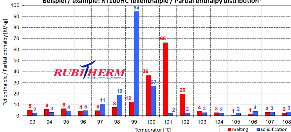
Beispiel / example: RT100HC Teilenthalpie / Partial enthalpy distribution*
