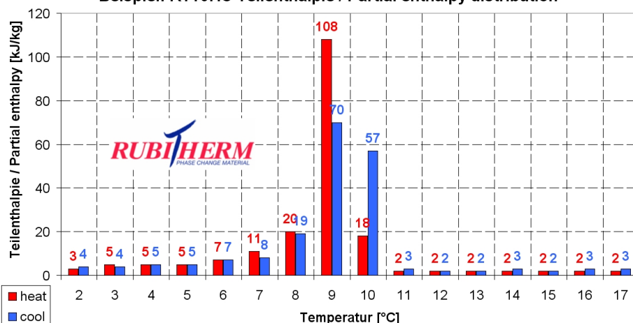
Beispiel: RT10HC Teilenthalpie / Partial enthalpy distribution
