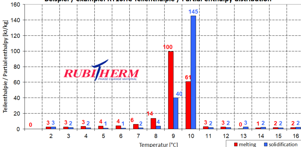
Beispiel / example: RT10HC Teilenthalpie / Partial enthalpy distribution
