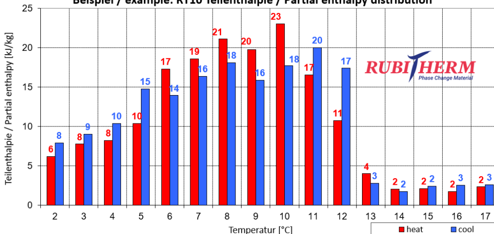
Beispiel / example: RT10 Teilenthalpie / Partial enthalpy distribution*
