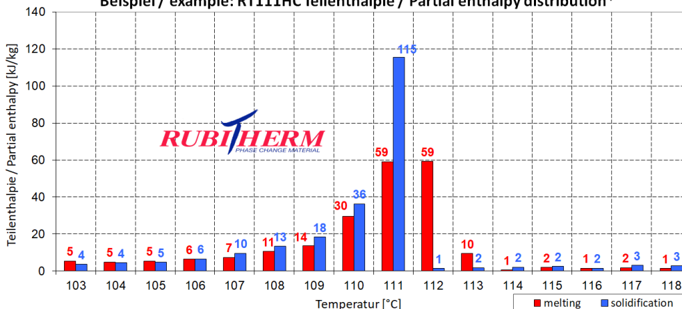
Beispiel / example: RT111HC Teilenthalpie / Partial enthalpy distribution*
