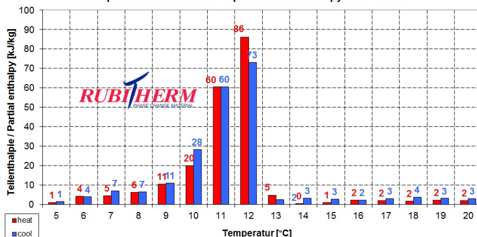
Beispiel: RT11HC Teilenthalpie / Partial enthalpy distribution
