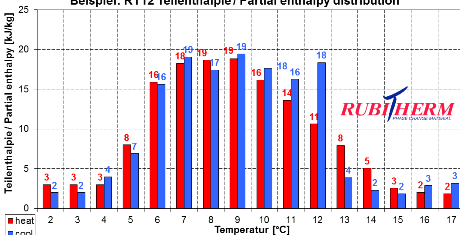
Beispiel: RT12 Teilenthalpie / Partial enthalpy distribution
