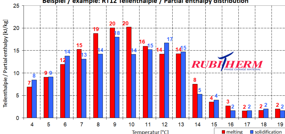
Beispiel / example: RT12 Teilenthalpie / Partial enthalpy distribution
