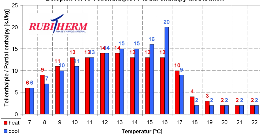
Beispiel: RT15 Teilenthalpie / Partial enthalpy distribution
