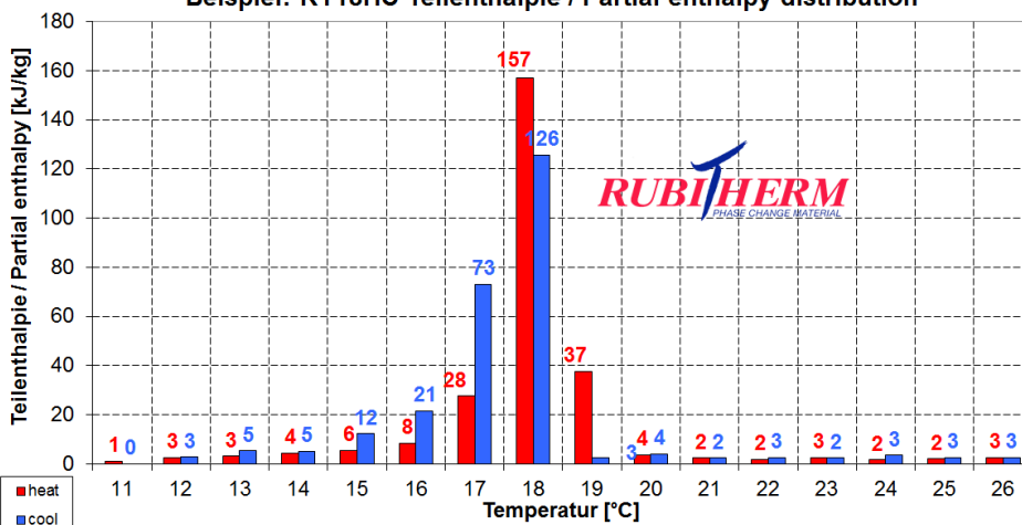
Beispiel: RT18HC Teilenthalpie / Partial enthalpy distribution
