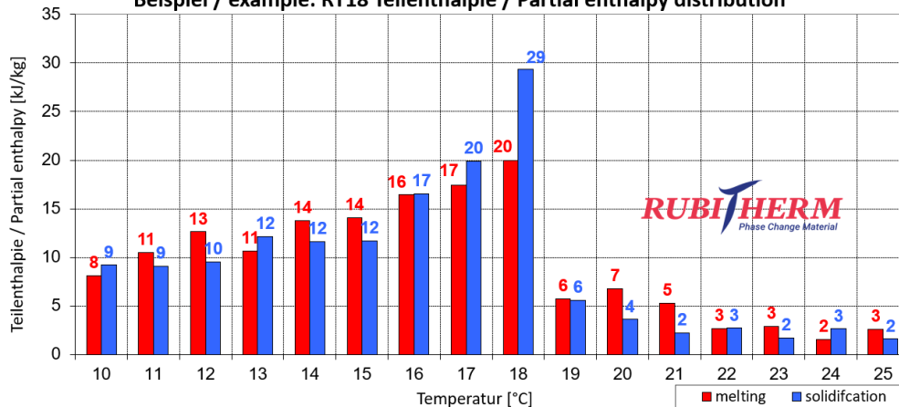
Beispiel / example: RT18 Teilenthalpie / Partial enthalpy distribution*
