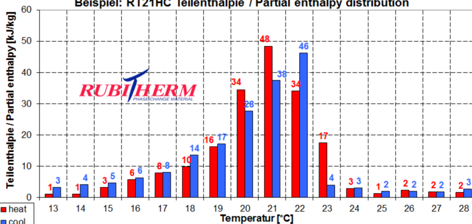
Beispiel: RT21HC Teilenthalpie / Partial enthalpy distribution
