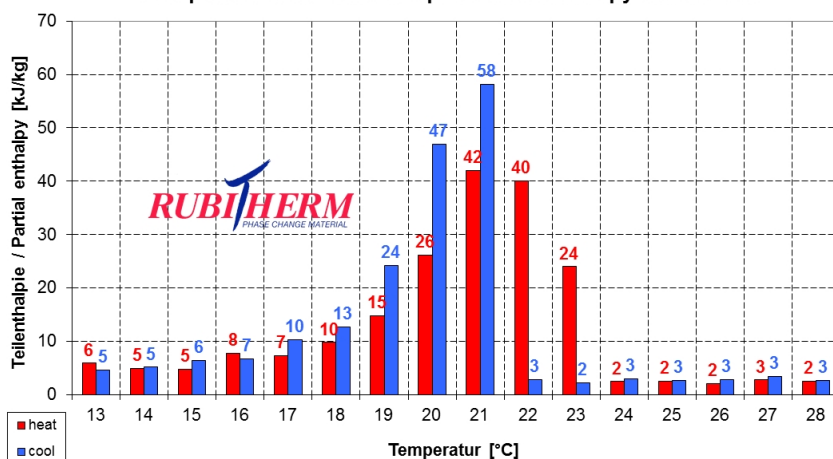
Beispiel: RT21HC Teilenthalpie / Partial enthalpy distribution
