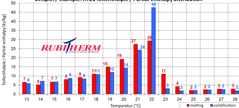
Beispiel / example: RT21 Teilenthalpie / Partial enthalpy distribution
