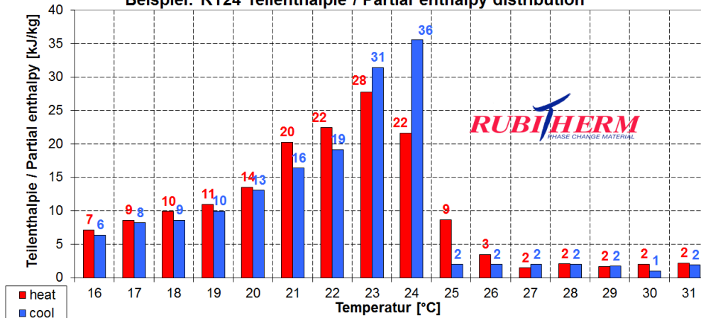
Beispiel: RT24 Teilenthalpie / Partial enthalpy distribution
