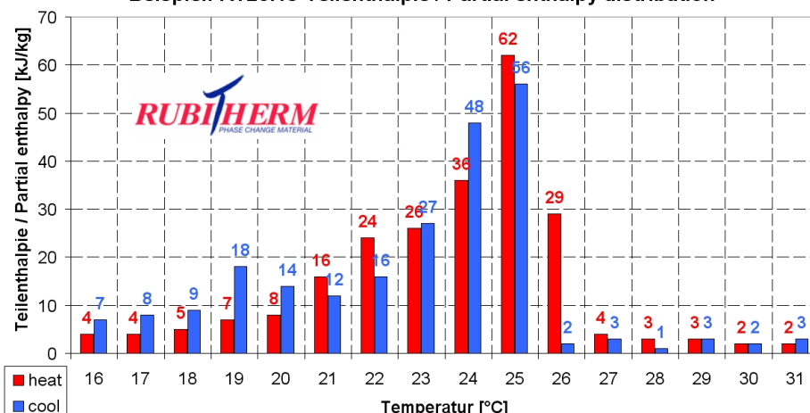
Beispiel: RT25HC Teilenthalpie / Partial enthalpy distribution
