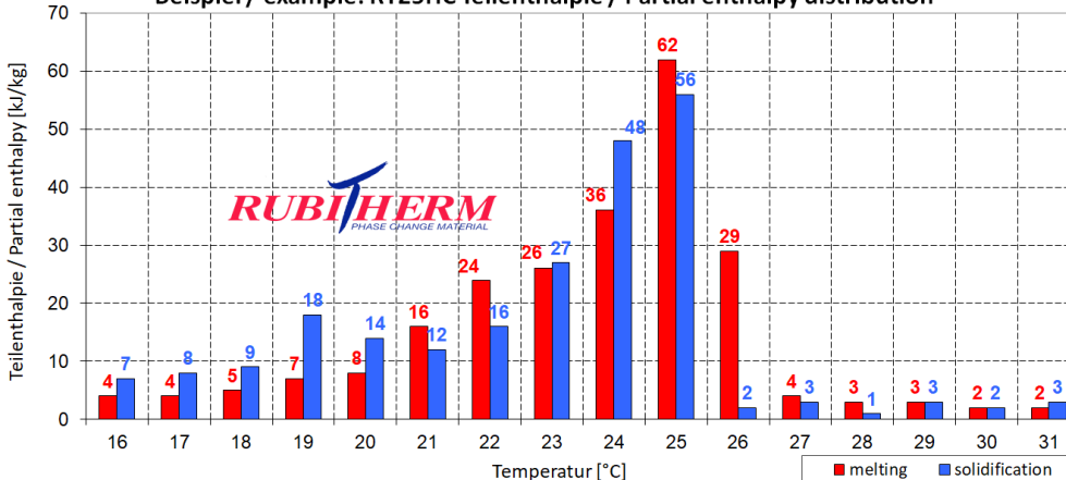
Beispiel / example: RT25HC Teilenthalpie / Partial enthalpy distribution
