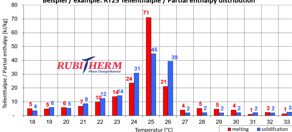
Beispiel / example: RT25 Teilenthalpie / Partial enthalpy distribution*
