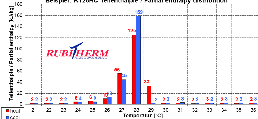
Beispiel: RT28HC Teilenthalpie / Partial enthalpy distribution
