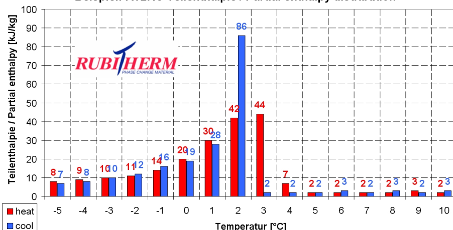
Beispiel: RT2HC Teilenthalpie / Partial enthalpy distribution
