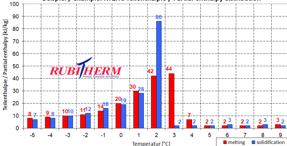
Beispiel / example: RT2HC Teilenthalpie / Partial enthalpy distribution
