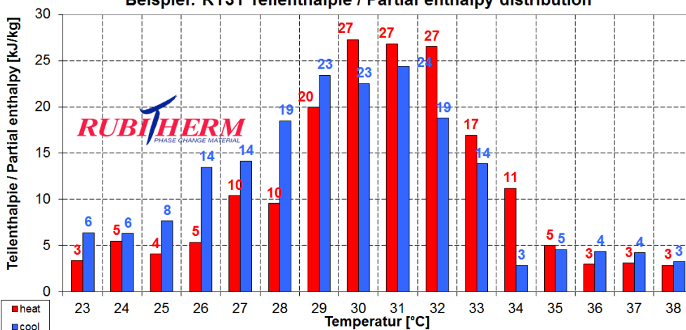
Beispiel: RT31 Teilenthalpie / Partial enthalpy distribution
