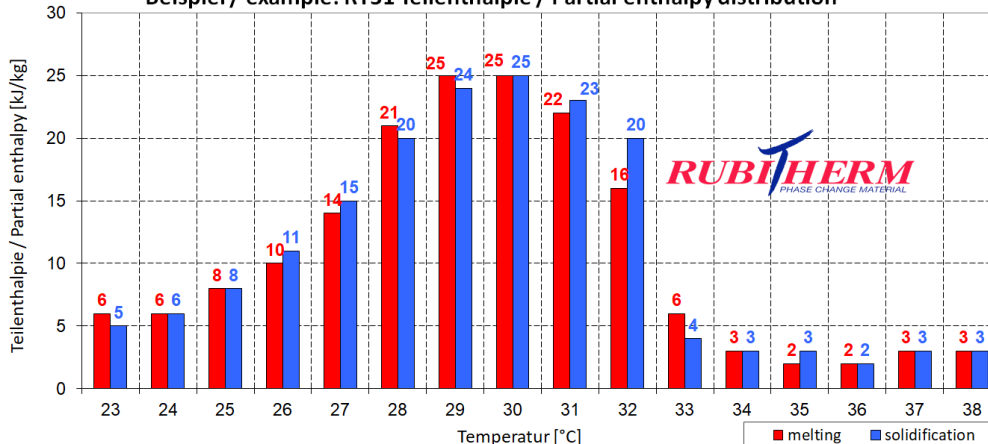
Beispiel / example: RT31 Teilenthalpie / Partial enthalpy distribution
