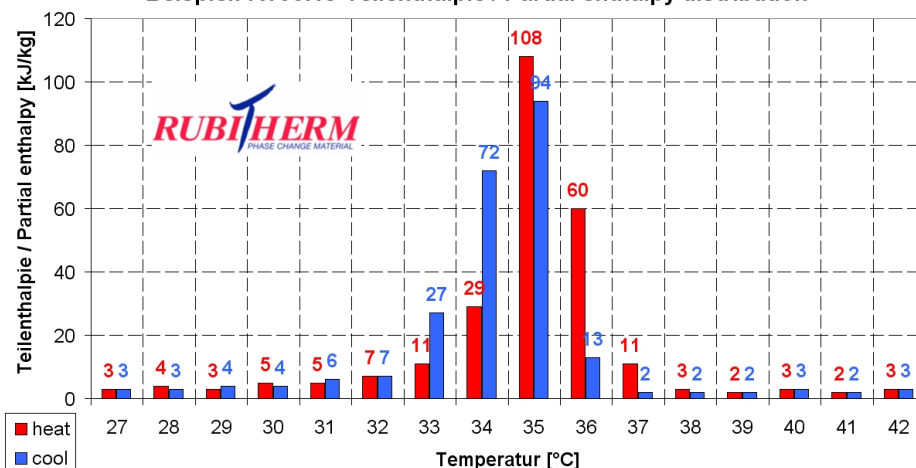
Beispiel: RT35HC Teilenthalpie / Partial enthalpy distribution
