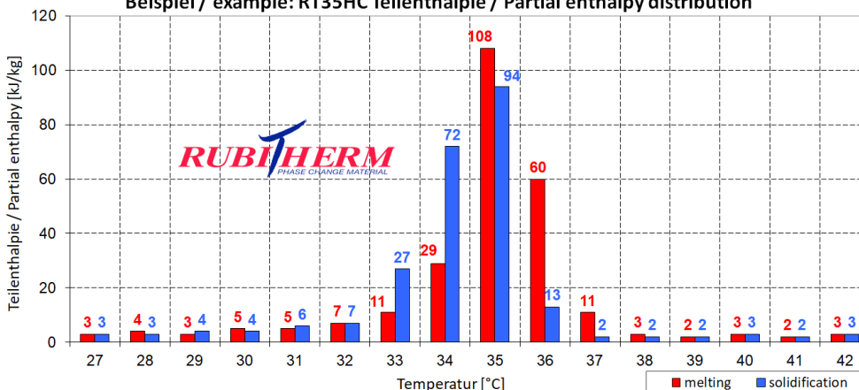
Beispiel / example: RT35HC Teilenthalpie / Partial enthalpy distribution
