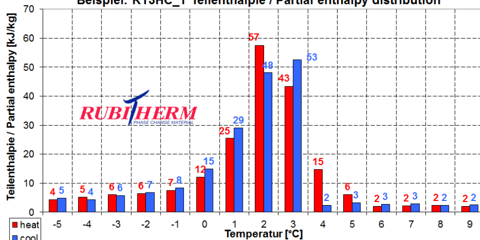
Beispiel: RT3HC_1 Teilenthalpie / Partial enthalpy distribution
