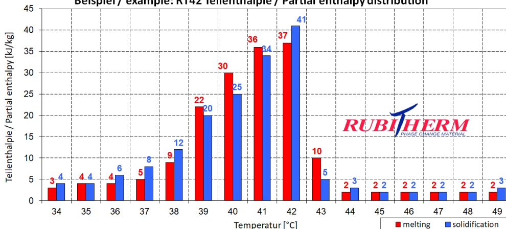
Beispiel / example: RT42 Teilenthalpie / Partial enthalpy distribution
