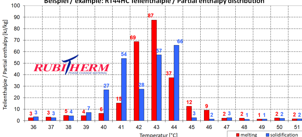
Beispiel / example: RT44HC Teilenthalpie / Partial enthalpy distribution
