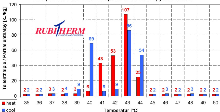
Beispiel: RT44HC Teilenthalpie / Partial enthalpy distribution
