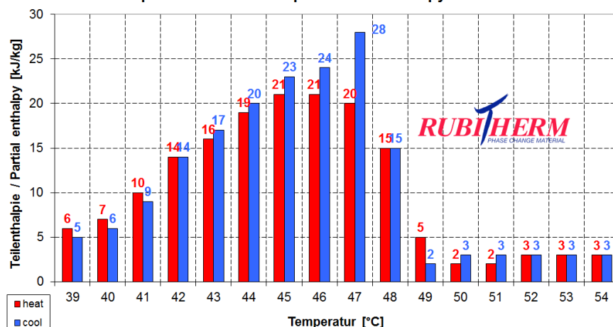
Beispiel: RT47 Teilenthalpie / Partial enthalpy distribution
