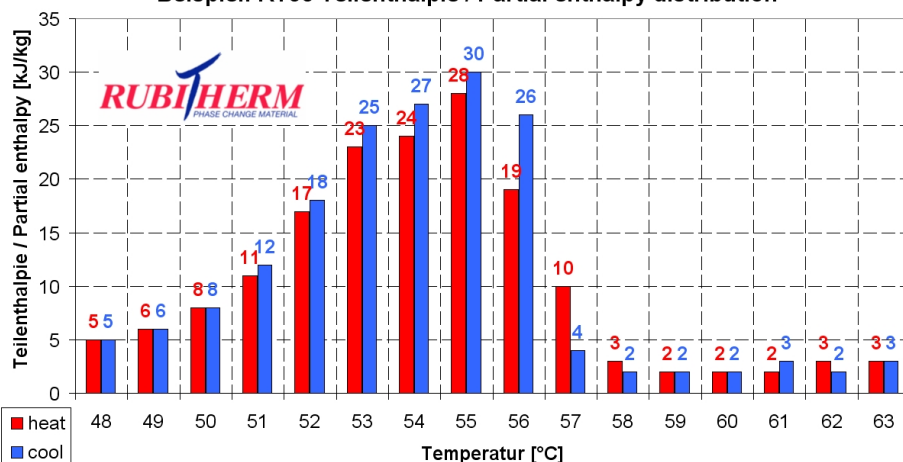
Beispiel: RT55 Teilenthalpie / Partial enthalpy distribution
