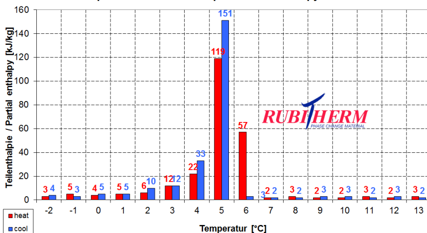
Beispiel: RT5HC Teilenthalpie / Partial enthalpy distribution
