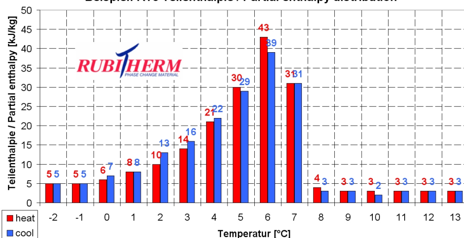
Beispiel: RT5 Teilenthalpie / Partial enthalpy distribution
