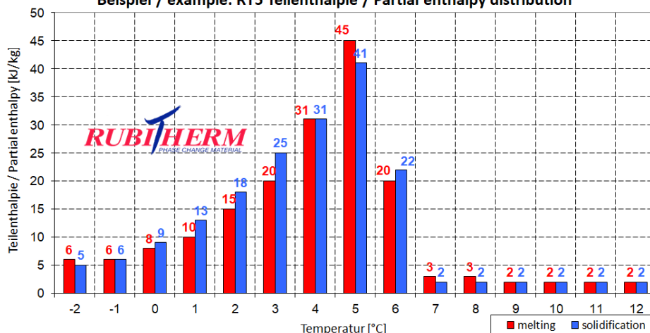
Beispiel / example: RT5 Teilenthalpie / Partial enthalpy distribution
