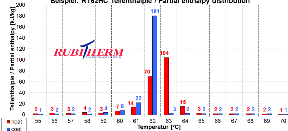
Beispiel: RT62HC Teilenthalpie / Partial enthalpy distribution
