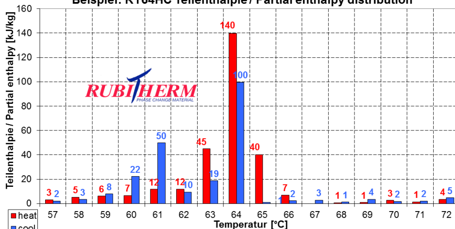
Beispiel: RT64HC Teilenthalpie / Partial enthalpy distribution
