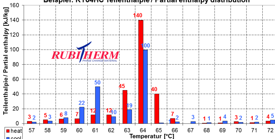
Beispiel: RT64HC Teilenthalpie / Partial enthalpy distribution
