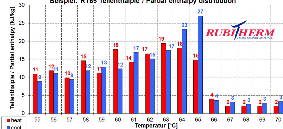
Beispiel: RT65 Teilenthalpie / Partial enthalpy distribution
