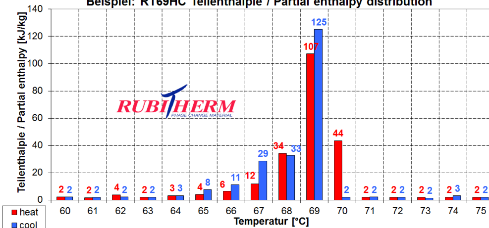
Beispiel: RT69HC Teilenthalpie / Partial enthalpy distribution
