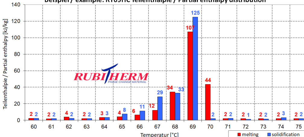
Beispiel / example: RT69HC Teilenthalpie / Partial enthalpy distribution*
