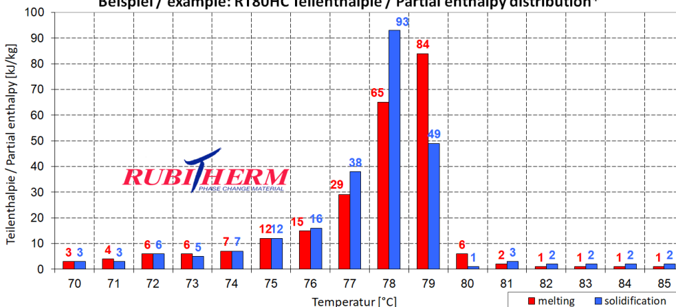
Beispiel / example: RT80HC Teilenthalpie / Partial enthalpy distribution*
