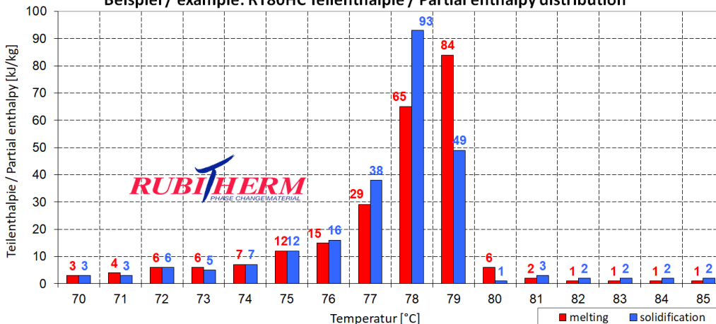
Beispiel / example: RT80HC Teilenthalpie / Partial enthalpy distribution*
