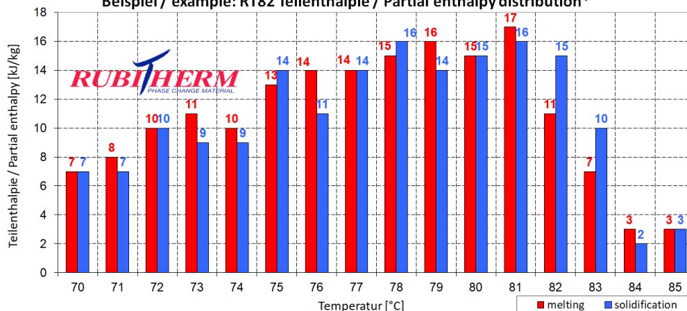
Beispiel / example: RT82 Teilenthalpie / Partial enthalpy distribution*
